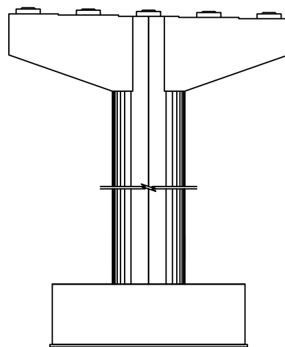
배면
