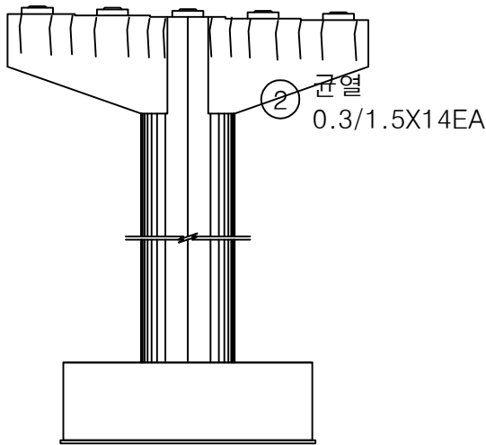
정면
