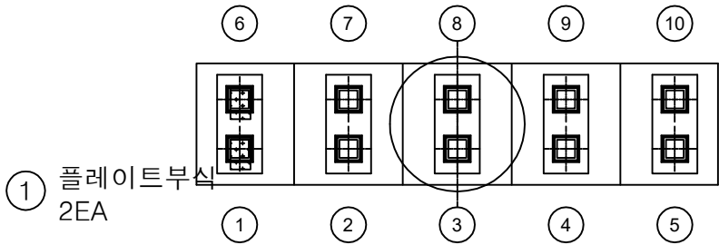
평면도
