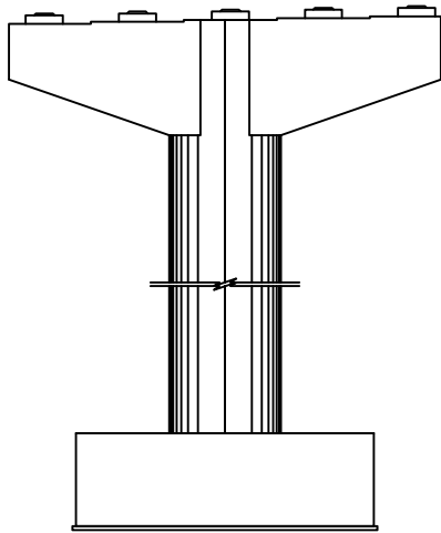
정면
