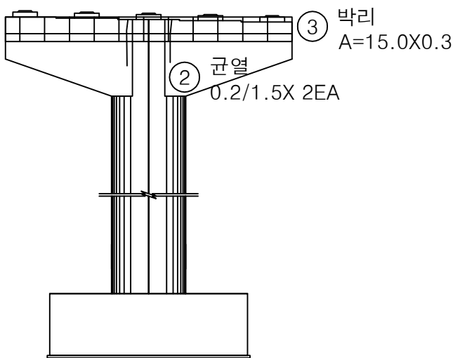
배면
