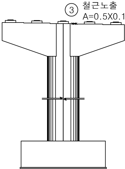
배면
