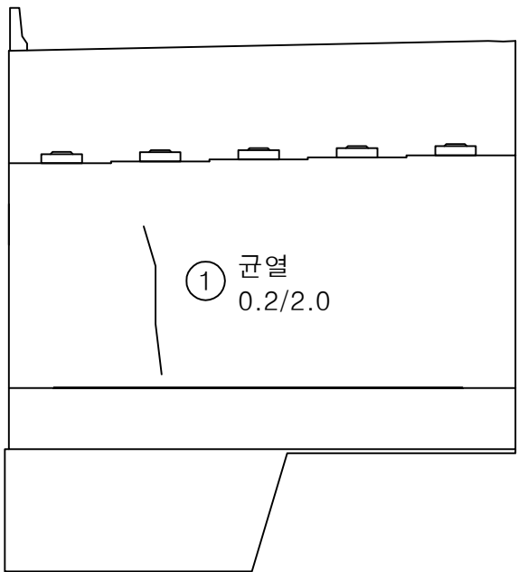
정면
