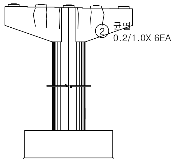
배면
